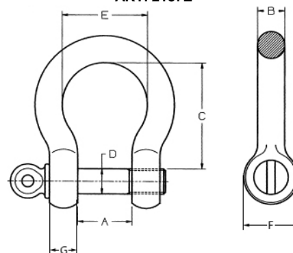
GRILLI AD OMEGA ZINCATI ART. 2157E
